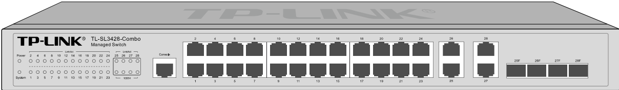
图 2-11 TL-SL3428-Combo 的前面板
