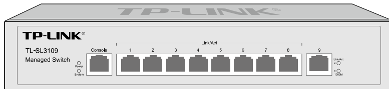
图 2-17 TL-SL3109 的前面板
