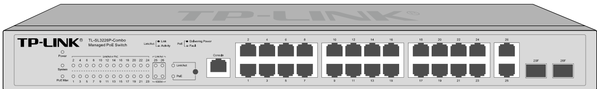
图 2-19 TL-SL3226P-Combo 的前面板
