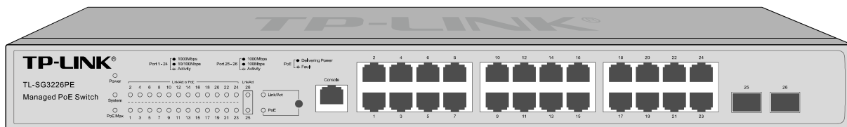
图 2-6 TL-SG3226PE 的前面板
