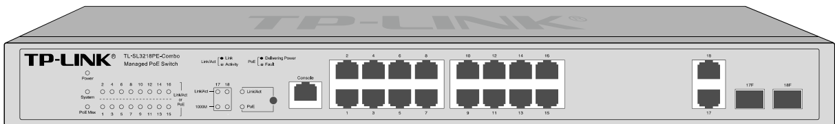
图 2-20 TL-SL3218PE-Combo 的前面板
