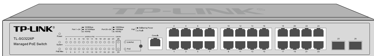
图 2-7 TL-SG3226P 的前面板
