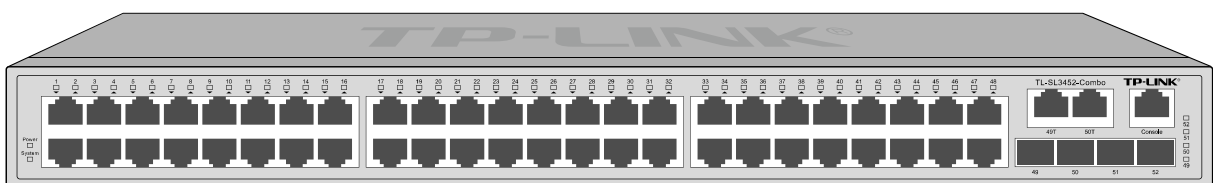
图 2-10 TL-SL3452-Combo 的前面板
