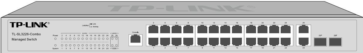
图 2-12 TL-SL3226-Combo 的前面板
