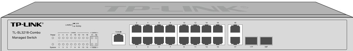
图 2-14 TL-SL3218-Combo 的前面板
